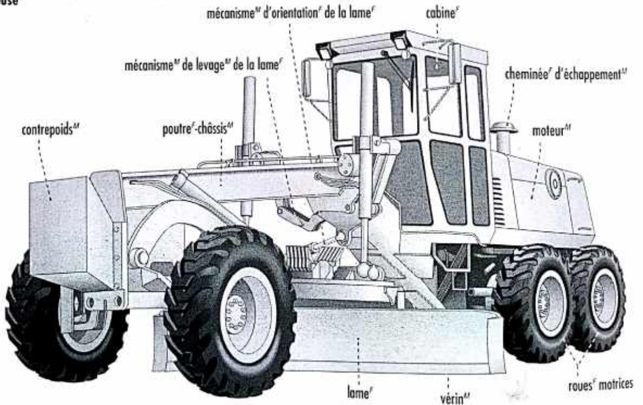
niveleuse f
