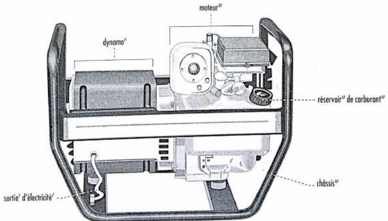
production F d'électricité F par groupe M électrogène
