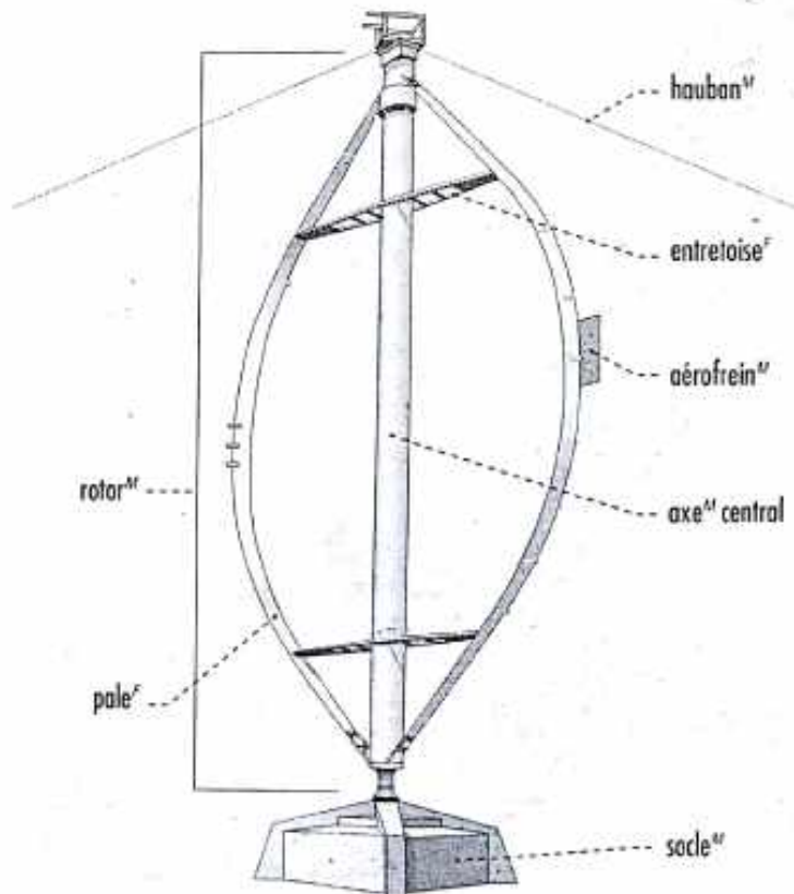
éolienne f à axe m vertical
