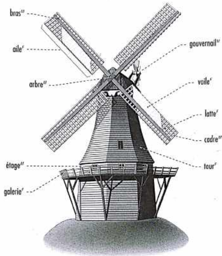
éolienne f à axe m horizontal
