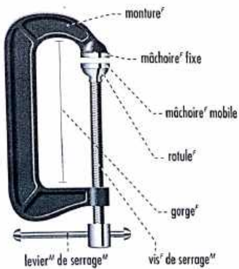
serre-joint
