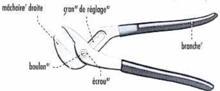
pince multiprise
