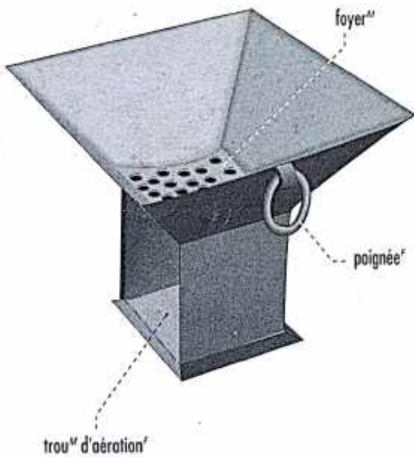
fourneau M malgache
