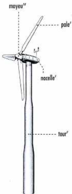
éolienne f à axe m horizontal
