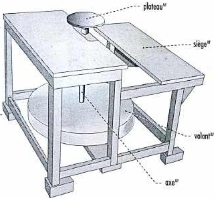
tour à pied
