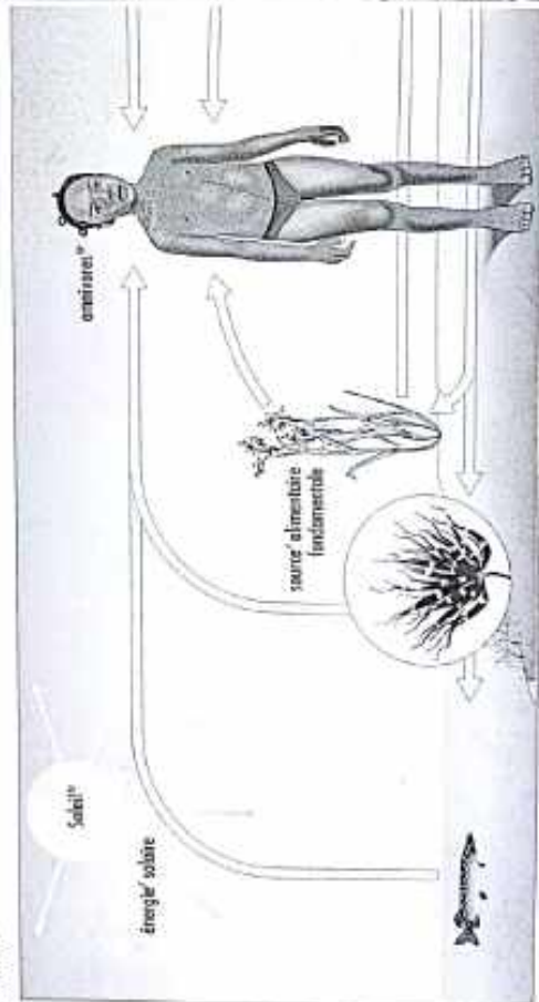
chaîne alimentaire
