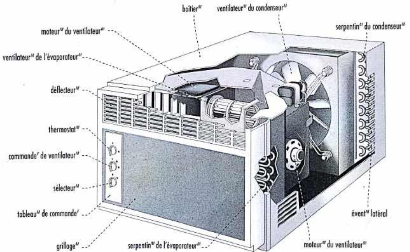
climatiseur m de fenêtre f
